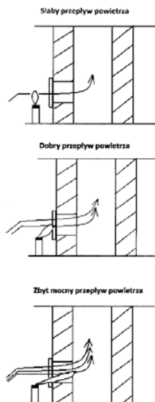
Rysunek nr 2: SPRAWDZENIE CIĄGU SPALINOWEGO
